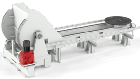
Vyklápěcí stůl pro stohy kol Bezpečné vyklápění a polohování stohovaných kol
