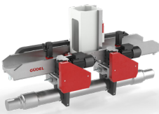
Chapadlo pro nápravy Bezpečná manipulace a boční zakládání železničních náprav; NC motoricky řízené jednoduché nebo dvojité nastavení rozteče
