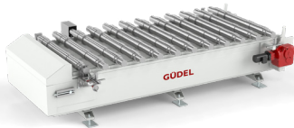
Kettenförderer für Achsen Zuverlässiger Transport von Eisenbahnachsen
