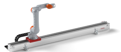
Bodenverfahrachse CoboMover CMF mit KUKA Cobot LBR iisy R1300
