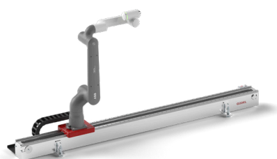
Axe linéaire au sol CoboMover CMF avec cobot ABB GoFa
